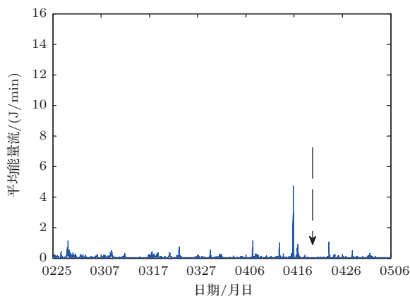
图10 2013年4月20日芦山7级地震前后异常次声波的短时能量曲线图
