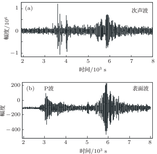
图 24 瑞士用次声传感器检测到的次声波和地震传感器检测到的地震信号
