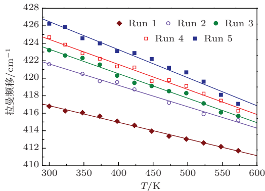
图7 (网刊彩色) 不同实验轮回下白宝石 \nu_{12} 拉曼峰随温度变化的关系
