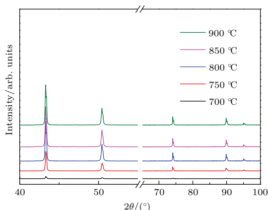
图6 (网刊彩色) 样品的 XRD 图
