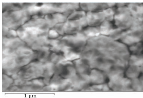
图5 在 900 °C 下制备的纳晶铜块体的 SEM 图
