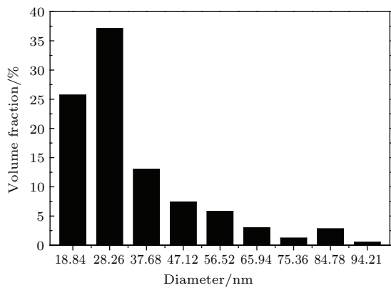
图1 纳米铜粉粒径的概率分布柱状图 Fig. 1. Statistical distribution of particle size.
