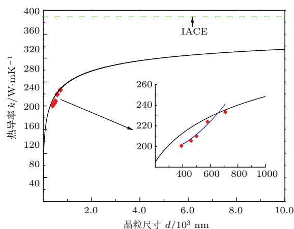
图8 (网刊彩色) 热导率与晶粒尺寸的关系
