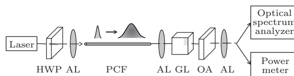
图6 装置示意图, 其中, HWP, 半波片; AL, 非球面透镜; PCF, 光子晶体光纤; GL, 格兰棱镜; OA, 光衰减器
