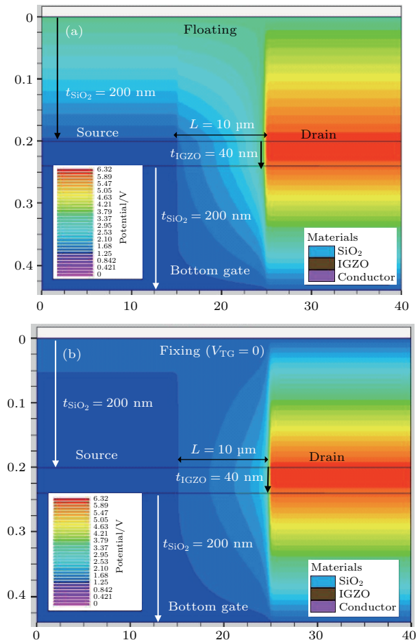
图2 (a)悬浮的, (b)固定电位的遮光金属栅IGZO TFT的电势分布剖面图( V_{\text{DS}} = 5 \text{ V} )
