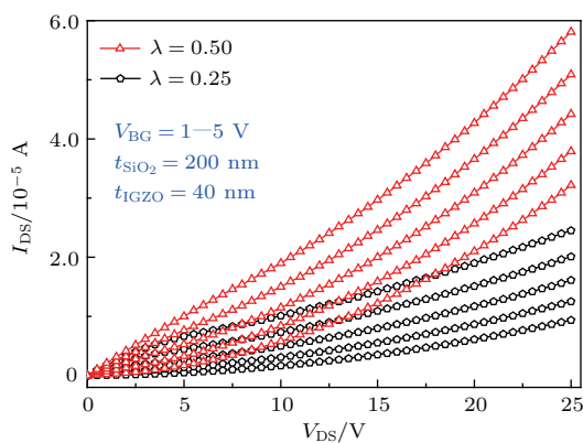
图8 遮光金属栅悬浮的IGZO TFT输出特性曲线在不同 \lambda 的取值下的模型计算值对比
