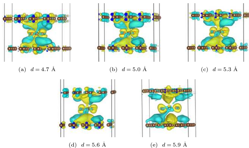
图5 CO与O反应,在不同间距的双层石墨烯间过渡态的电荷差分密度图,其中等值面数值分别为 (a) 0.00014 e (a.u.) 3 ; (b) 0.00020 e (a.u.) 3 ; (c) 0.00025 e (a.u.) 3 ; (d) 0.00035 e (a.u.) 3 ; (e) 0.00048 e (a.u.) 3
