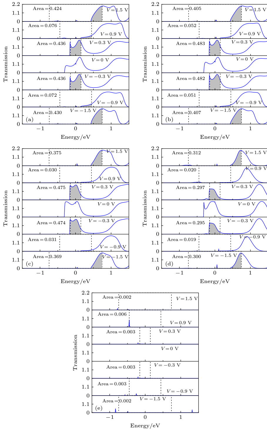
图 5 偏压 0, \pm 0.3 V, \pm 0.9 V 以及 \pm 1.5 V 下喹啉 C_9H_5N 分子平面与石墨烯纳米带电极分别成 (a) 0^\circ , (b) 30^\circ , (c) 45^\circ , (d) 60^\circ 和 (e) 90^\circ 时的透射谱, 图中的黑色虚线和阴影部分面积分别表示偏压窗和偏压窗内透射系数积分面积
