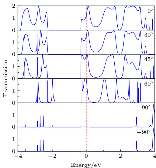
图 6 零偏压下, 喹啉 C_9H_5N 分子平面与石墨烯纳米带电极成 0^\circ , 30^\circ , 45^\circ , 60^\circ , 90^\circ 和 -90^\circ 角度下的透射谱, 其中红色虚线表示费米能级
