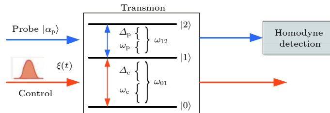
图 2 基于单 transmon 的微波光子探测系统
