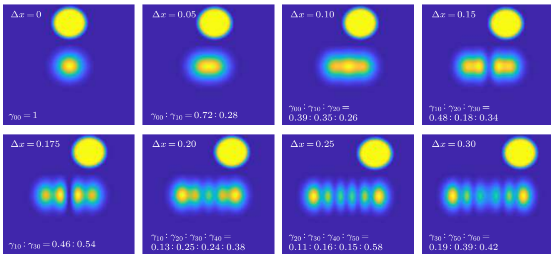
图 5 抽运功率 0.5 W、抽运光半径 0.15 mm 时, 8 个离轴量下的光斑
