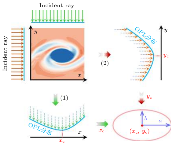
图 4 计算涡核位置坐标的原理图
