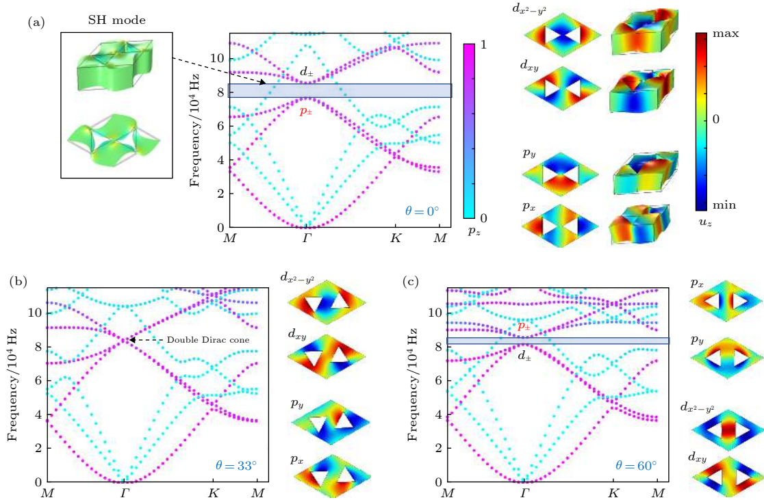
图 2 三角形穿孔声子晶体板在不同旋转角度下的能带结构与本征态 z 方向位移场分布 (a) \theta = 0^\circ , p_{\pm} 模位于 d_{\pm} 模下方, 左侧插图图 2(a) 左侧插图为 P_z = 0 点所对应的水平剪切模振型, 右侧插图为 p_{\pm} 和 d_{\pm} 模态的位移场分布和振型, 能带结构中用不同颜色表示 P_z 极化指标; (b) \theta = 33^\circ , 偶然简并形成双狄拉克锥, 右侧插图图 2(b) 右侧插图为 p_{\pm} 和 d_{\pm} 模态的位移场分布; (c) \theta = 60^\circ , p_{\pm} 模位于 d_{\pm} 模上方
