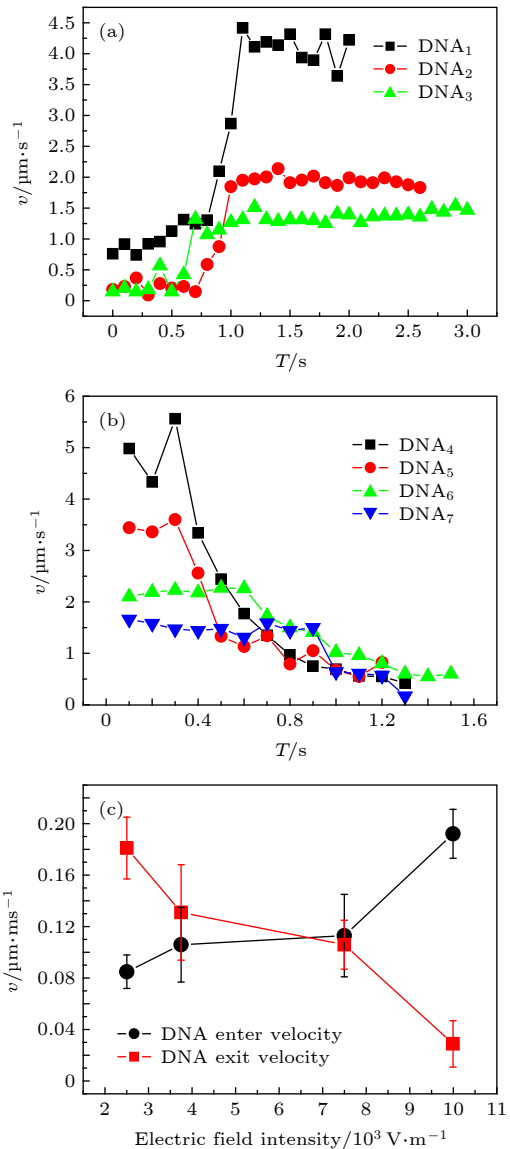
图 3 DNA 分子进出端口的速度随时间的变化 ( E = 3.75 \times 10^4 \text{ V}\cdot\text{m}^{-1} ) (a) 进入 trans 端口; (b) 穿出 cis 端口; (c) 速度随外加电场强度的变化关系
