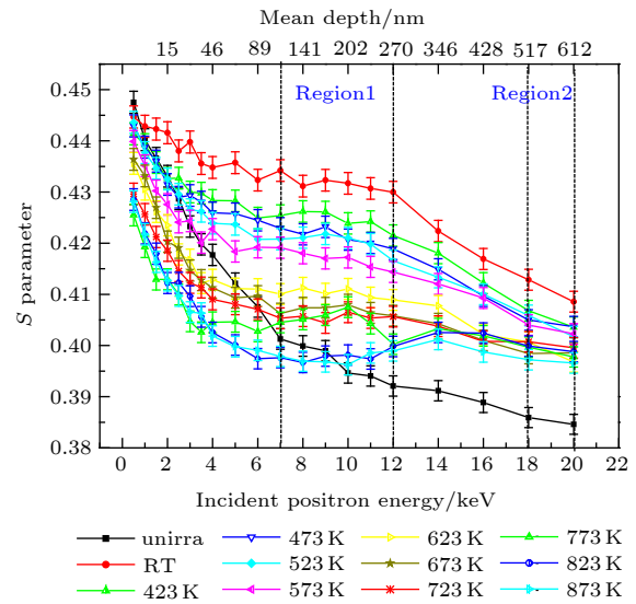
图7 氢辐照 Fe17Cr14.5Ni 等时退火过程 S - E 曲线随温度变化过程 [34]
