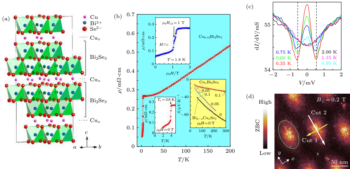
图 7 \text{Cu}_x\text{Bi}_2\text{Se}_3 中的非常规超导 (a) 能够发生超导相变的层间 Cu 掺杂 \text{Bi}_2\text{Se}_3 结构示意图 [81] ; (b) 输运测得的 \text{Cu}_{0.12}\text{Bi}_2\text{Se}_3 超导在电阻率-温度 ( \rho-T ) 关系中的反映, 左下角插图是超导转变区的放大, 上方插图是超导转变中电阻率随垂直于面的磁场强度的关系, 右下方插图是不同掺杂方式和比例的样品 Seebeck 系数随温度的关系, 说明了填隙方式掺入 Cu 有更好的掺杂效果 [81] ; (c) 在点接触谱中观察到的 \text{Cu}_x\text{Bi}_2\text{Se}_3 超导的 ZBCP [90] ; (d) STM 观测到的 \text{Cu}_{0.31}\text{Bi}_2\text{Se}_3 在电子温度 310 mK 和 0.2 T 的垂直磁场下磁通涡旋中的 ZBCP [84] .
