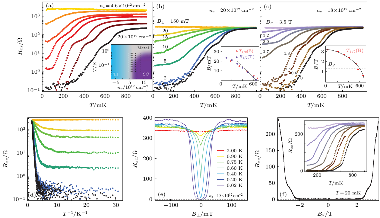
图3 Sajadi等 [63] 的WTe 2 栅压实验 (a) 零外磁场下,不同载流子浓度下的 \ln R_{xx}-T 曲线,其中出现明显的中间态平台.插图为扫描线在相图中的位置;(b)载流子浓度 n_e = 20 \times 10^{12} \text{ cm}^{-2} 时,不同垂直场下的 \ln R_{xx}-T 曲线.插图:扫温得到的特征温度 T_{1/2} 和扫场得到特征磁场 B_{1/2} ;(c)载流子浓度 n_e = 18 \times 10^{12} \text{ cm}^{-2} 时,不同平行场下的 \ln R_{xx}-T 曲线( B_{//} = 0 数据对应载流子浓度 n_e = 19 \times 10^{12} \text{ cm}^{-2} ;剩余数据对应载流子浓度 n_e = 18 \times 10^{12} \text{ cm}^{-2} ).插图:特征温度 T_{1/2} 随平行场 B_{//} 的变化关系,其中泡利极限 B_P 由灰色虚线表示;(d)不同垂直磁场下的 \ln R_{xx}-1/T 曲线,体现低温下电阻的饱和;(e)载流子浓度 n_e = 15 \times 10^{12} \text{ cm}^{-2} 时,不同温度下的 R_{xx}-B_{\perp} 曲线体现极低垂直磁场下电阻的升高;(f)和(e)相同载流子浓度下,不同温度下的 R_{xx}-B_{//} 曲线,体现相比(e)更为尖锐的电阻跳变.插图:线性坐标下(c)中的数据.引自文献 [63]
