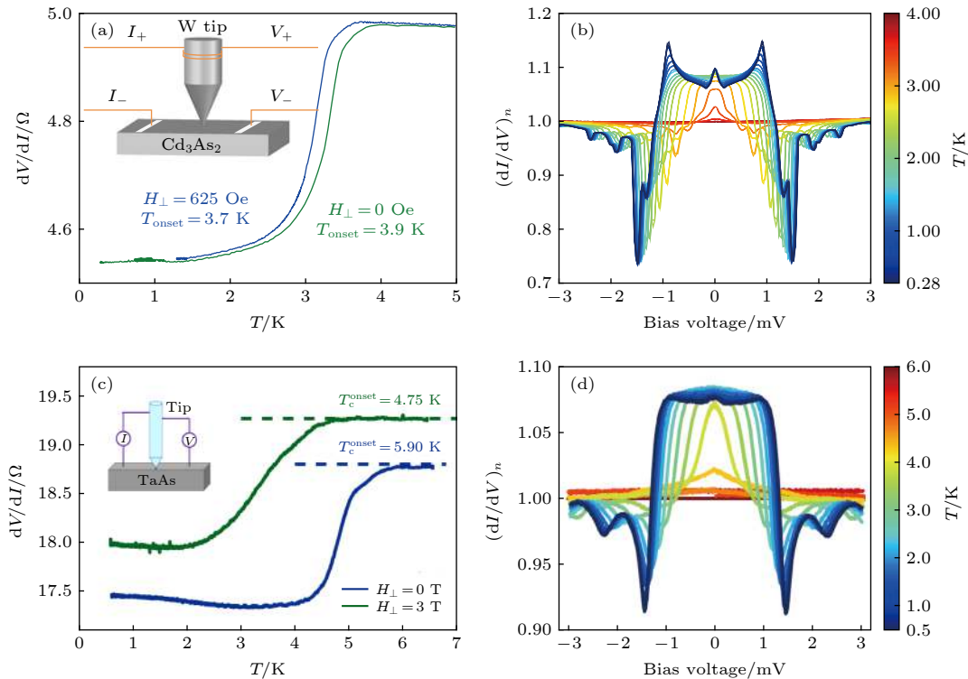
图 12 针尖点接触在拓扑半金属 \text{Cd}_3\text{As}_2 和 TaAs 中诱导的超导 (a) \text{Cd}_3\text{As}_2 中零偏压点接触微分电阻与温度的关系, 电阻的下降可以被磁场抑制, 这意味着它代表超导相变, 插图是针尖点接触实验装置示意图 [121]; (b) 不同温度下归一化的钨针尖 \text{Cd}_3\text{As}_2 点接触微分电导谱 [121]; (c), (d) PtIr 针尖点接触在 TaAs 中测得的超导 [123]
