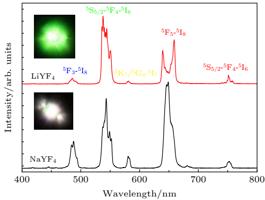
图4 在980 nm 激光激发下,单颗NaYF 4 :20.0%Yb 3+ /2.0%Ho 3+ 微米晶体和LiYF 4 :20.0%Yb 3+ /2.0%Ho 3+ 微米晶体的上转换发射光谱图(激发功率为100 mW/cm 2 )
