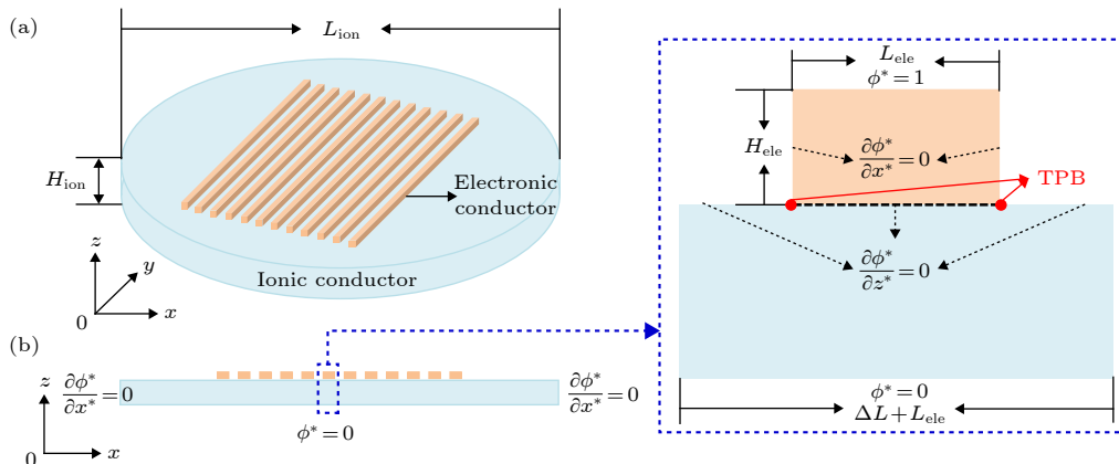
图 1 (a) 模式阳极结构示意图; (b) 本文计算区域与边界条件
