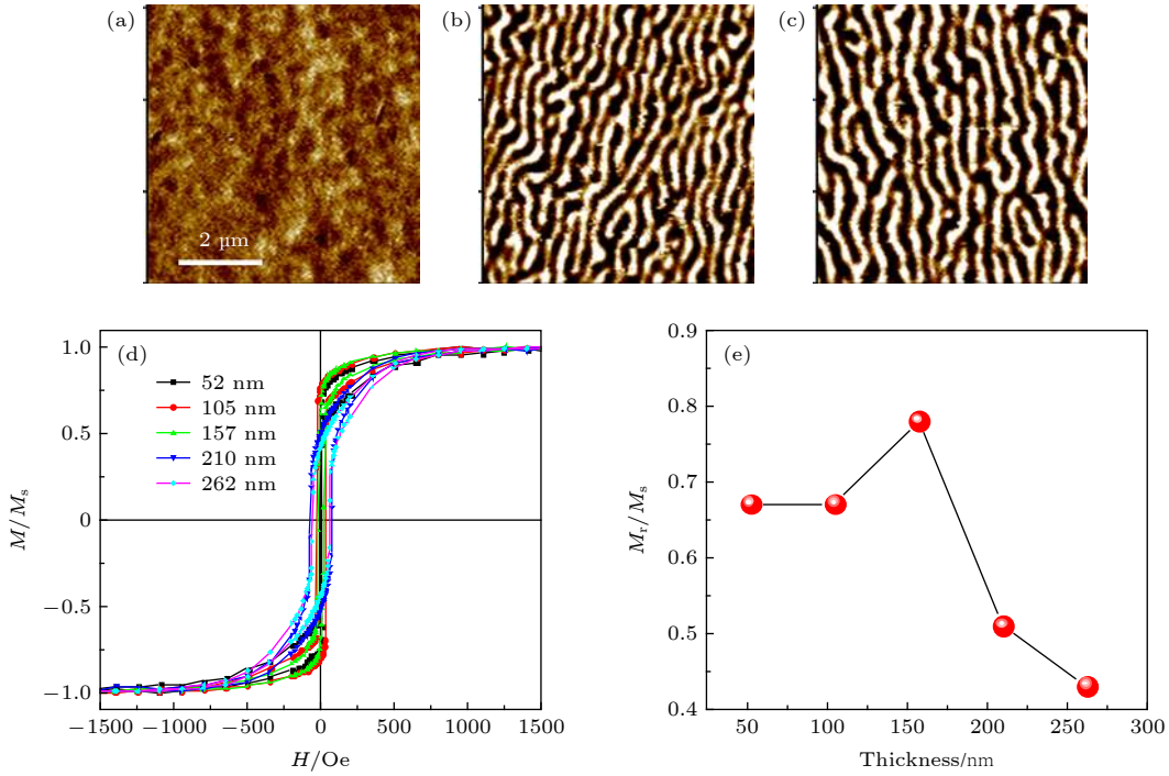
图 2 未进行热处理的膜厚为 (a) 105 nm, (b) 210 nm 和 (c) 262 nm 的 Ni 88 Cu 12 薄膜的 MFM 图像; (d) 不同厚度 Ni 88 Cu 12 薄膜的面内归一化磁滞回线; (e) 薄膜的 M_r/M_s 随薄膜厚度的变化 Fig. 2. The MFM images of (a) 105 nm, (b) 210 nm and (c) 262 nm-thick Ni 88 Cu 12 films before heat treatment; (d) in-plane normalized hysteresis loop of Ni 88 Cu 12 ; (e) remanence ratio vs. film thickness.
