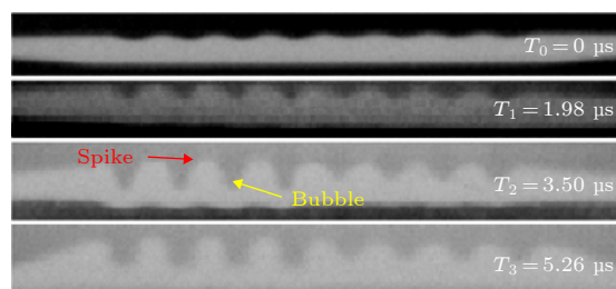
图 3 不同时刻界面扰动增长的 X 光图像
