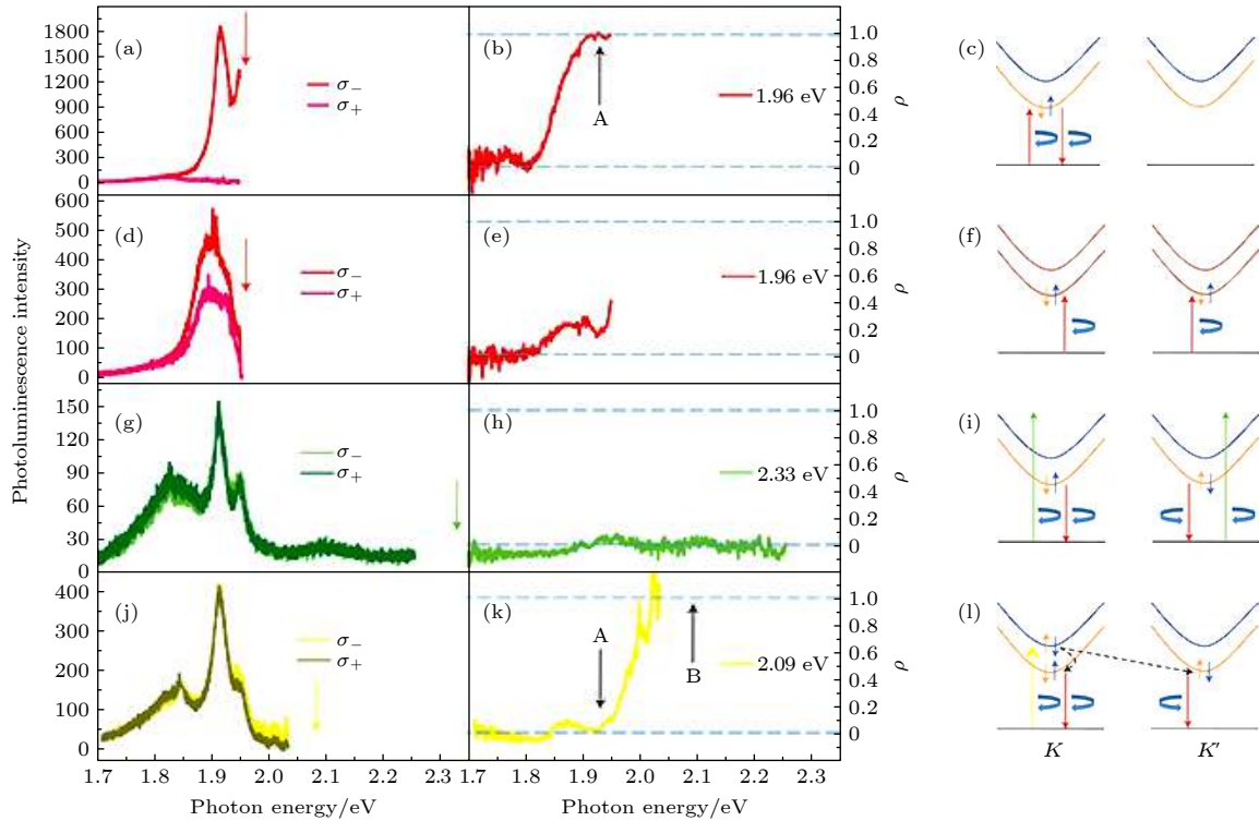
图9 光控制单层 MoS 2 的谷自旋极化 [49] (a)–(c) 单层 MoS 2 在 1.96 eV (633 nm) 激发, A 激子共振; (d)–(f) 1.96 eV 时双层 MoS 2 的激发; (g)–(i) 在 2.33 eV (532 nm) 下激发单层, 与 A, B 激子均非共振; (j)–(l) 在 2.09 eV (594 nm) 下激发单层, 与 B 激子共振. 左列: \sigma^- 和 \sigma^+ 分辨光致发光光谱. 中间柱: 相应的光致发光极化率作为光子能量的函数. 右柱: 光学吸收和发射过程的示意图
