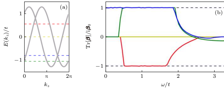
图 7 两带模型 Weyl 半金属的量子化的 CPGE 效应 [48] (a) 两带 Weyl 半金属模型的能带结构; (b) 在图 (a) 虚线所示四个化学势下 CPGE 张量的迹
