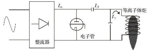
图 2 射频电源电路框图
