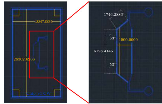
图 A1 微流控芯片沟道设计 CAD 图及设计参数
