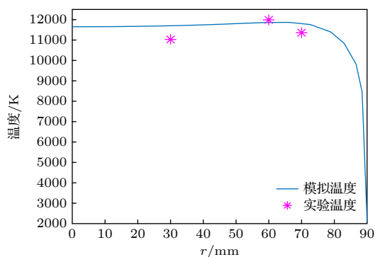
图 16 仿真温度与实验温度对比图
