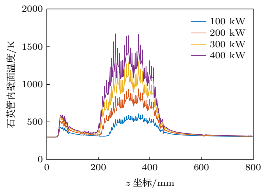
图 9 不同功率下石英管内壁面的温度分布
