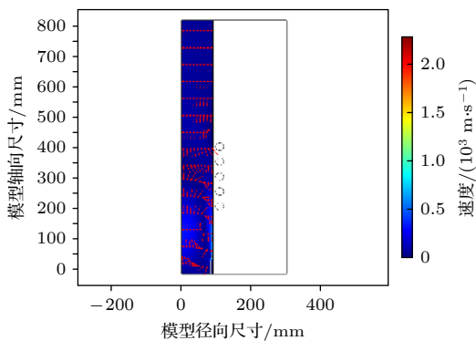
图 7 400 kW 等离子体速度分布
