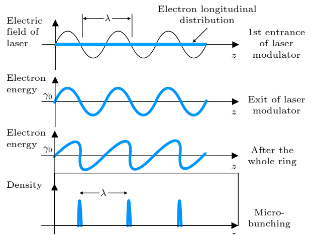
图 3 微聚束的原理示意图 Fig. 3. Schematic of the microbunching mechanism.
