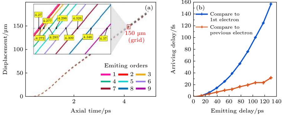
图 5 (a) 电子随时间的位移, 位移为 150 \mu\text{m} (栅极) 的区域展示于嵌入图中; (b) 电子到达栅极的相对延迟
