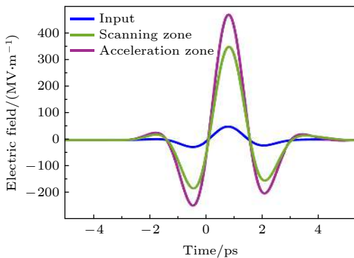
图 3 太赫兹脉冲输入波形、以及在加速腔和扫描腔中心处的波形
