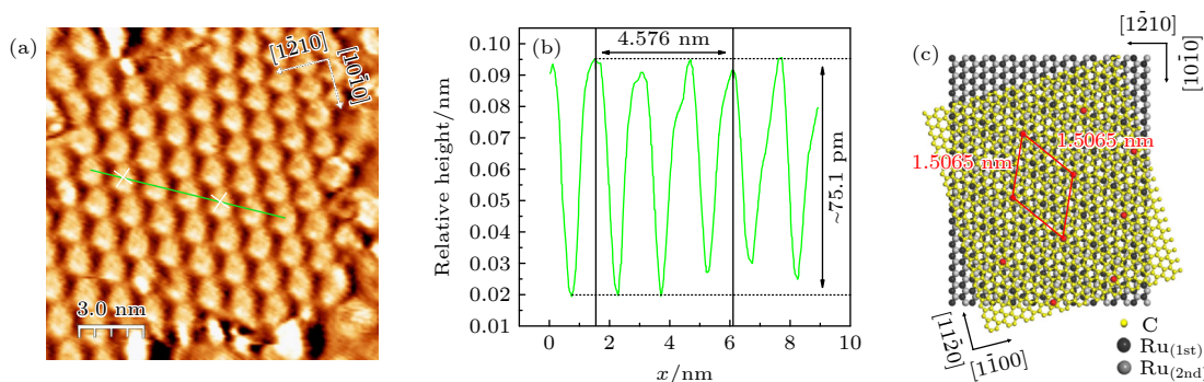
图 6 (a) 图 4(a) 中黄框区域的摩尔超结构图 ( 16.1^\circ 的摩尔超结构) ( 15 \text{ nm} \times 15 \text{ nm} , V_T = -0.401 \text{ V} , I_T = 0.258 \text{ nA} ); (b) 图 (a) 中沿着绿线的高度分布图; (c) 石墨烯与 Ru(0001) 衬底成 16.1^\circ 夹角的摩尔超结构模拟图 (其中黑色圆球代表衬底第一层钌原子, 灰色圆球代表衬底第二层钌原子, 黄色部分为石墨烯)
