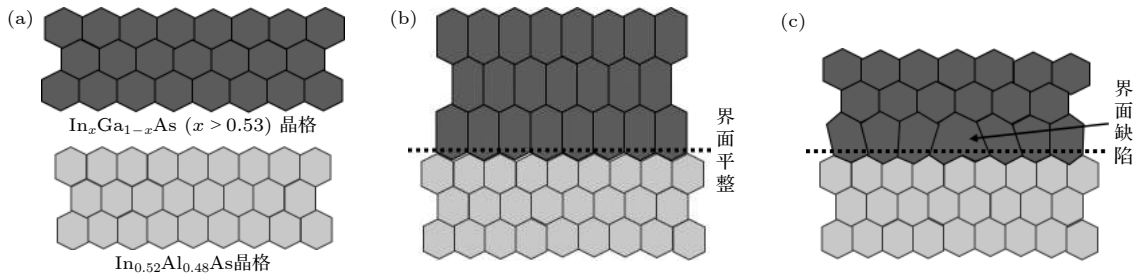
图 7 InGaAs/InAlAs 应变异质结的外延生长及弛豫示意图 (a) 两种不同晶格常数外延层; (b) 应变异质结; (c) 弛豫异质结
