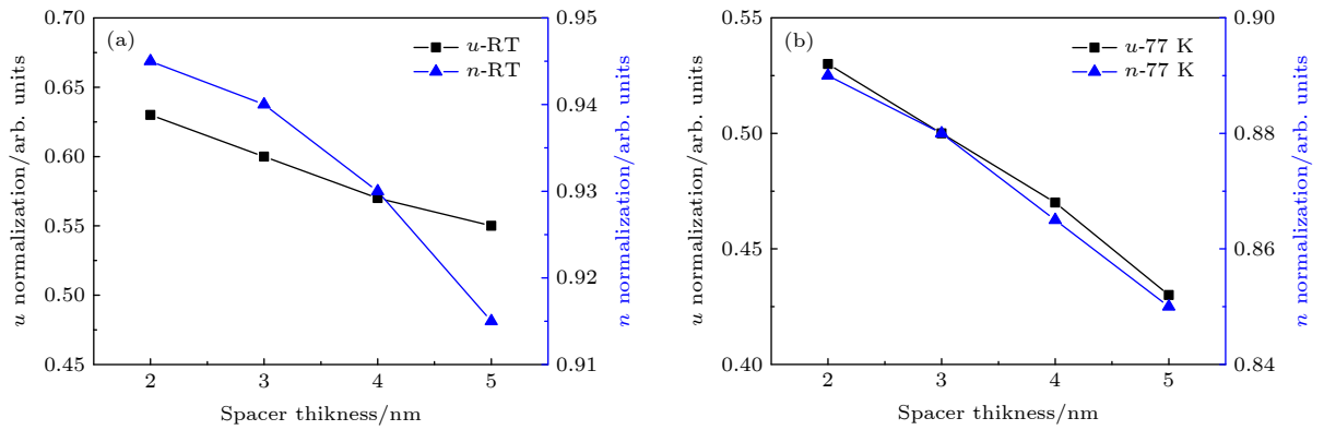
图 4 电子辐照对不同隔离层厚度 InP HEMT 二维电子气浓度和电子迁移率的归一化影响 (a) 室温; (b) 77 K
