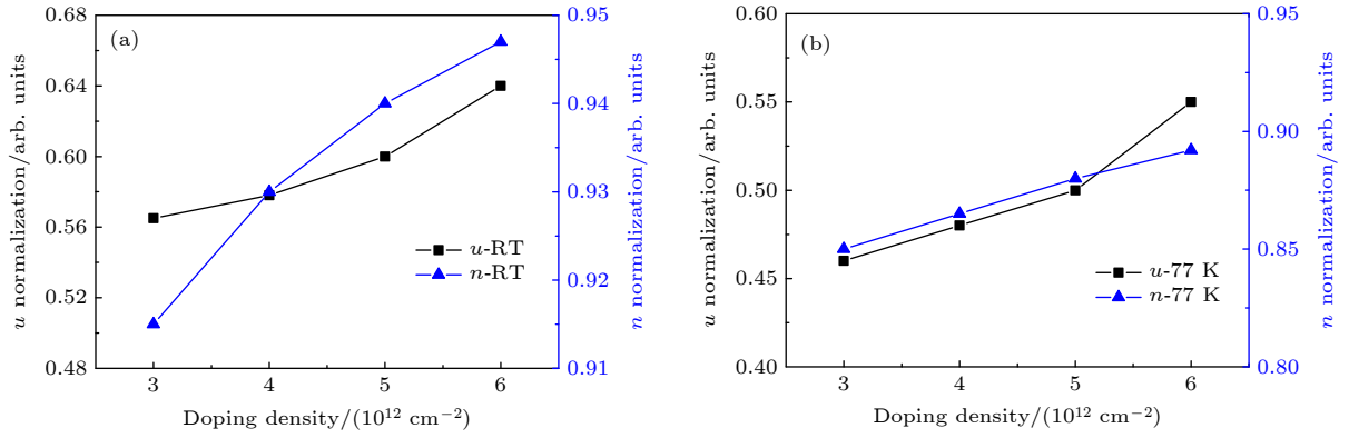
图 3 电子辐照对不同 \delta 掺杂浓度 InP HEMT 二维电子气浓度和电子迁移率的归一化影响 (a) 室温; (b) 77 K
