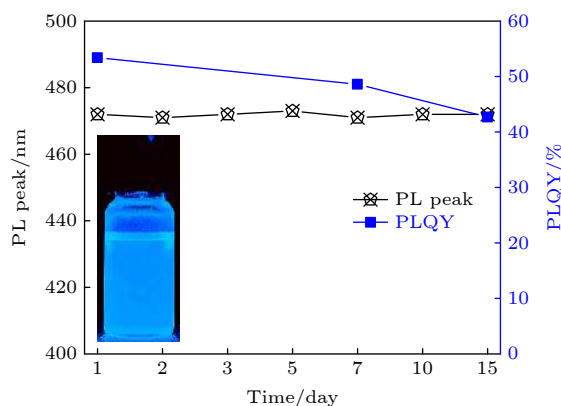
图 7 锡离子掺杂 \text{CsPbBr}_3 量子点大气氛围存放 1—15 d 的荧光峰位置及 PLQY 变化
