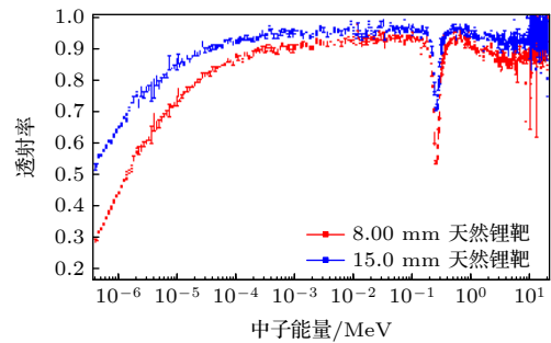
图 6 测得的天然锂样品的中子透射率
