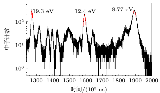
图4 裂变层第1层 235 U共振裂变峰的高斯拟合
