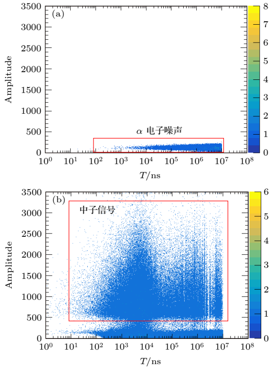
图2 第一层 235 U裂变层时间-幅度二维谱 (a) 无束流空靶; (b) 有束流空靶
