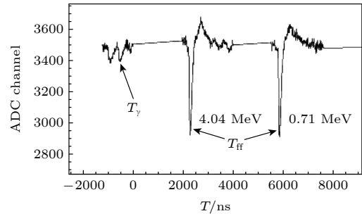
图3 裂变室输出的时间信号示例
