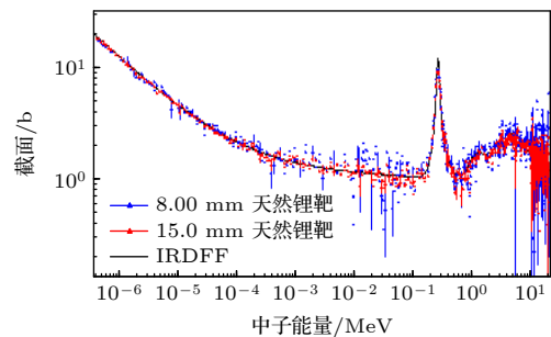
图 7 实验测得的天然锂中子全截面数据与 IRDF 评价数据库中的数据 (1 b = 10 -28 m 2 )
