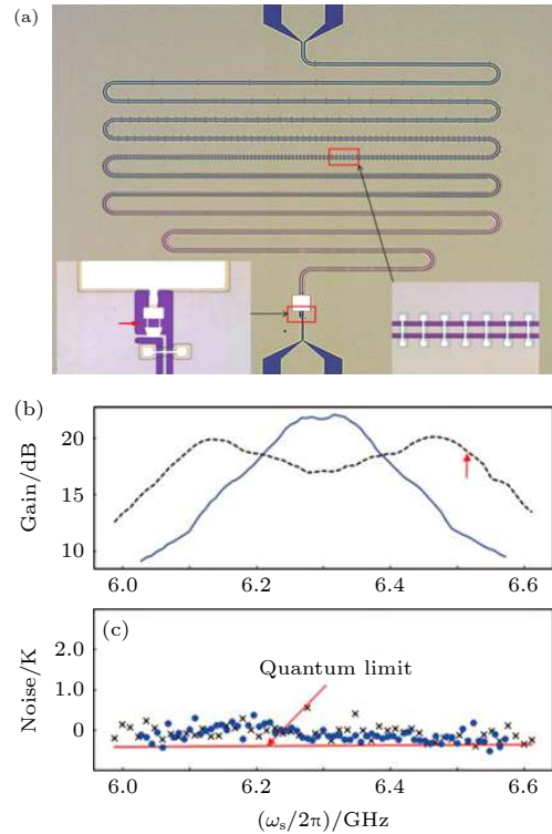
图 10 (a) 铌基 JPA 光学照片; (b) 增益与 (c) 噪声温度随频率的关系 [41]
