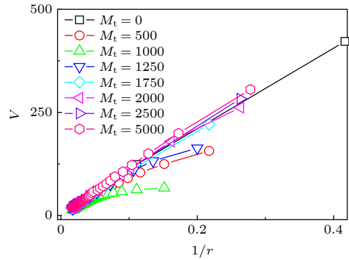
图 4 不同 M_t 条件下晶界迁移速率 ( V ) 与晶界半径倒数 ( 1/r ) 间的关系曲线 Fig. 4. The grain boundary migration velocity ( V ) versus the grain boundary curvature ( 1/r ) with different M_t .
