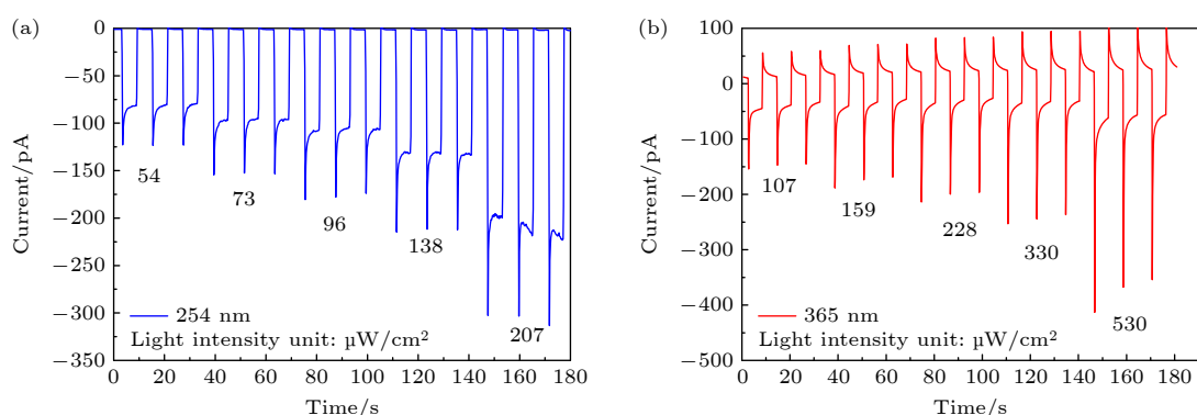
图4 零偏压下 (a) 254 nm 波长紫外光照射下的对数 I - t 特性曲线; (b) 365 nm 波长紫外光照射下的对数 I - t 特性曲线 Fig. 4. The I - t curves under (a) 254 nm and (b) 365 nm light illumination at zero bias.
