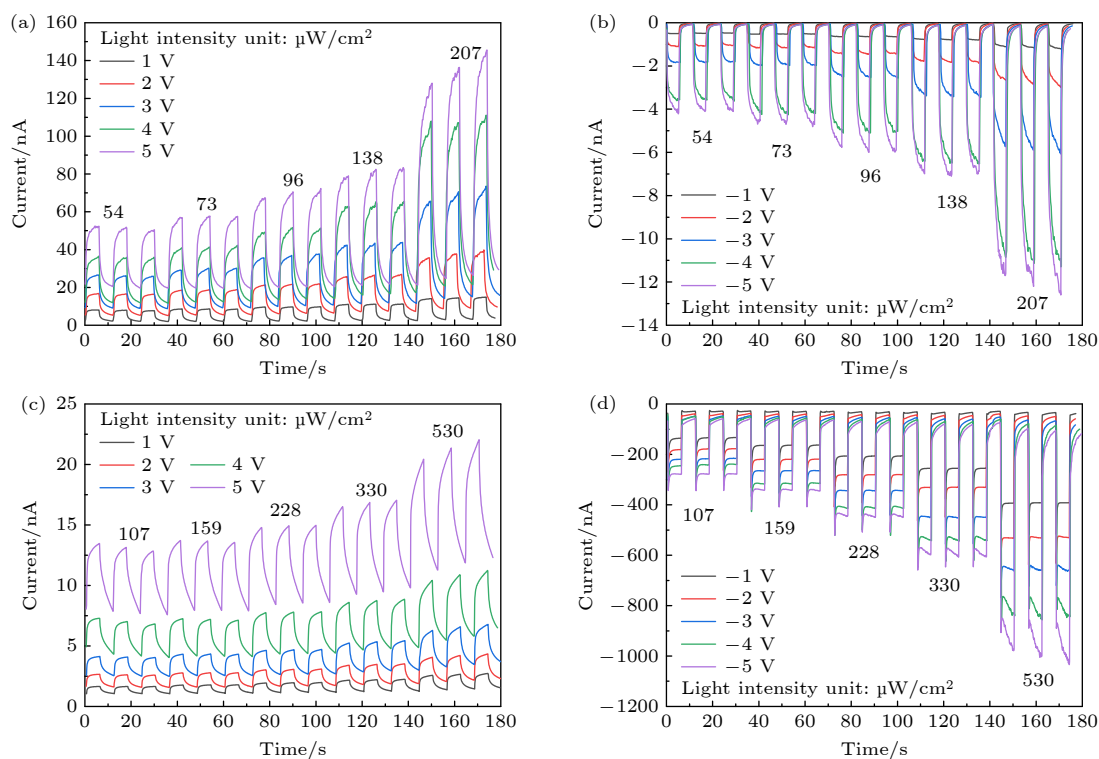
图5 (a) 正向偏压下、(b) 反向偏压下 254 nm 波长光辐照下的 I - t 特性曲线; (c) 正向偏压下、(d) 反向偏压下 365 nm 波长光辐照下的 I - t 特性曲线
