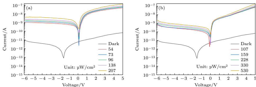
图 3 \text{Ga}_2\text{O}_3/\text{Al}_{0.1}\text{Ga}_{0.9}\text{N} 异质结光电探测器的对数形式的 I - V 特性曲线 (a) 暗条件与 254 nm 波长紫外光辐照; (b) 暗条件与 365 nm 波长紫外光辐照
