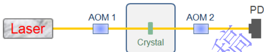
图2 实验装置的示意图。激光器输出的580 nm激光被一个声光调制器（AOM1）所调制，并入射到低温系统内的晶体样品(Crystal)上。输出光场被另一个声光调制器（AOM2）所调制，最终由探测器探测（PD）。
