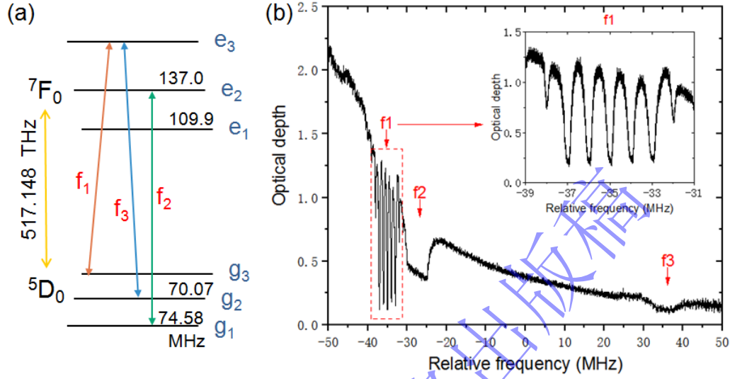
图4 (a) ^{153}\text{Eu}^{3+} 离子能级结构。(b)在偏离中心频率位置上制备的AFC结构，其频率中心为517.14873 THz。(b)中插图放大AFC光谱结构。
