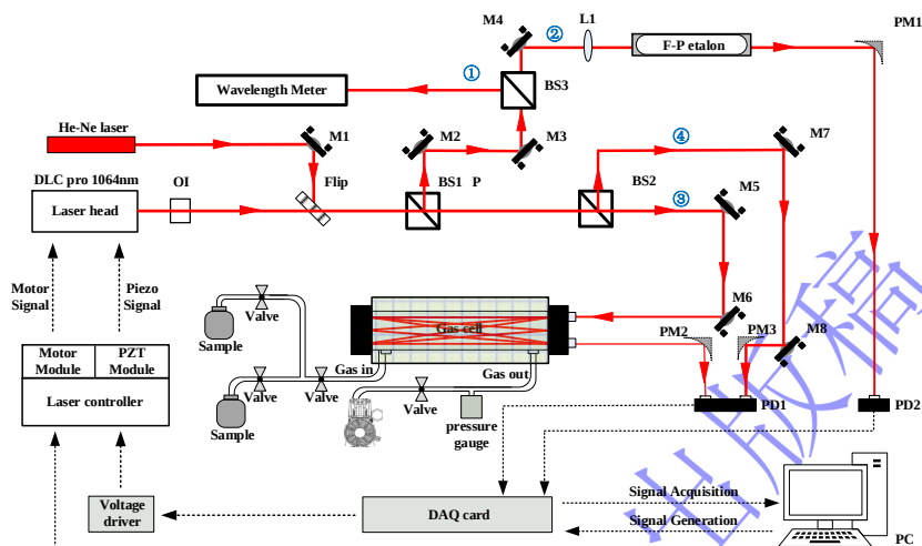
图 1 水分子吸收光谱实验装置
