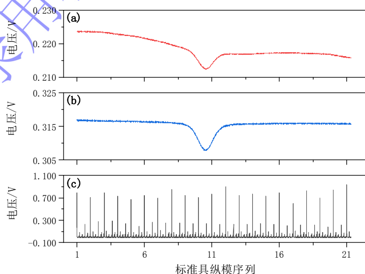
图 2 吸收信号对比 (a) 光束 4 引入前获得的水分子吸收信号；
