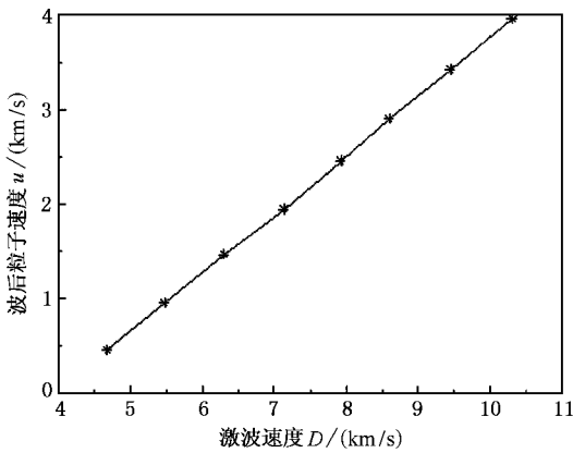
图2 冲击波速度 D 与波后粒子速度 u 关系图
