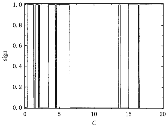
图 9 v = 1.0, \omega = 2.0, A = 10 粒子自俘获时相互作用强度 c 的临界值, sign = 1 表示粒子发生了自俘获, sign = 0 表示没发生自俘获. 图线跃变处即粒子自俘获时 c 的临界值
