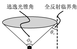
图2 逃逸光锥示意图
