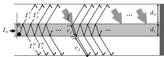
图3 光波导中荧光传输过程的示意图
