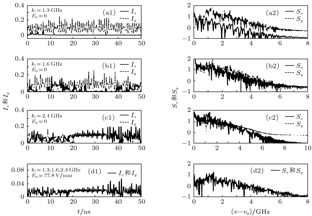
图 8 当 L = 10 \text{ mm} , \mu = 1.1 , 在不同 k_f 和 E_0 条件下, VCSEL 输出的偏振混沌的时间演变 (图左) 和对应的频谱分布 (图右). (a1, a2) E_0 = 0 \text{ V/mm} , k_f = 1.3 \text{ GHz} ; (b1, b2) E_0 = 0 \text{ V/mm} , k_f = 1.6 \text{ GHz} ; (c1, c2) E_0 = 0 \text{ V/mm} , k_f = 2.4 \text{ GHz} ; (d1, d2) E_0 = 77.8 \text{ V/mm} , k_f = 1.3, 1.6, 2.4 \text{ GHz}
