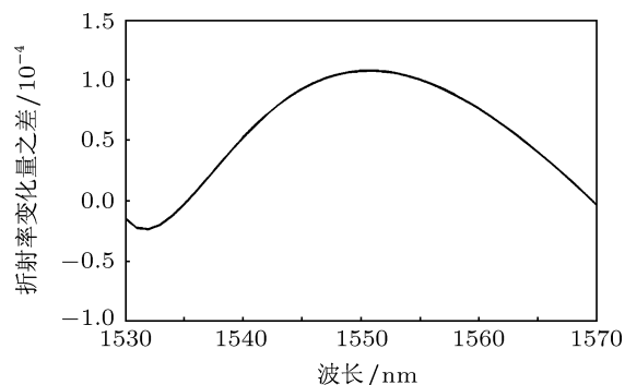
图 6 TE 模和 TM 模折射率变化量之差的波长响应谱
