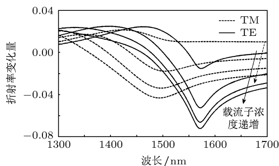
图 1 不同载流子浓度对应的 InGaAs/InGaAsP 量子阱结构折射率变化谱. 图中 TE (TM) 模曲线对应的载流子浓度由 1 \times 10^{18} \text{ cm}^{-3} 增加到 4 \times 10^{18} \text{ cm}^{-3} , 间隔为 1 \times 10^{18} \text{ cm}^{-3}
