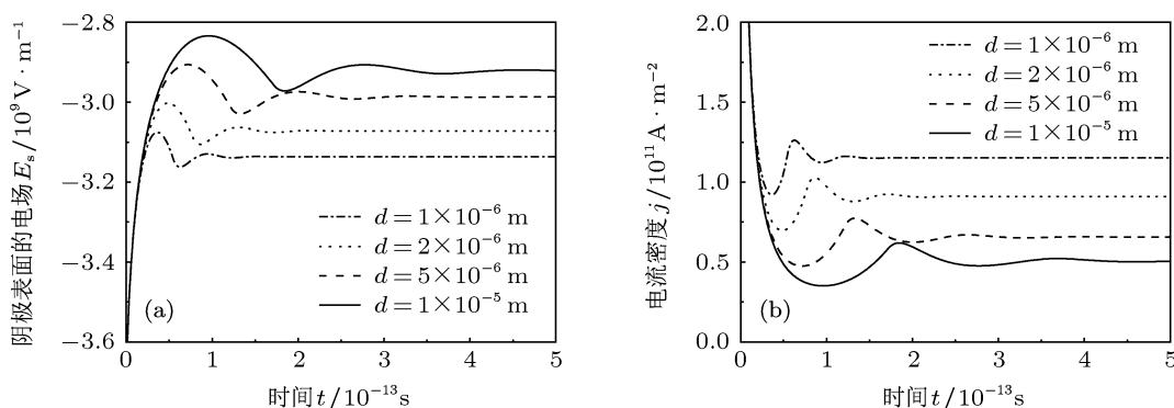
图 4 外加电场强度 E = -3.62 \times 10^9 \text{ V/m} 的结果 (a) 阴极表面电场随时间的变化; (b) 阴极发射电流密度随时间的变化
