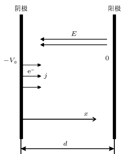
图 1 平板二极管几何模型示意图
