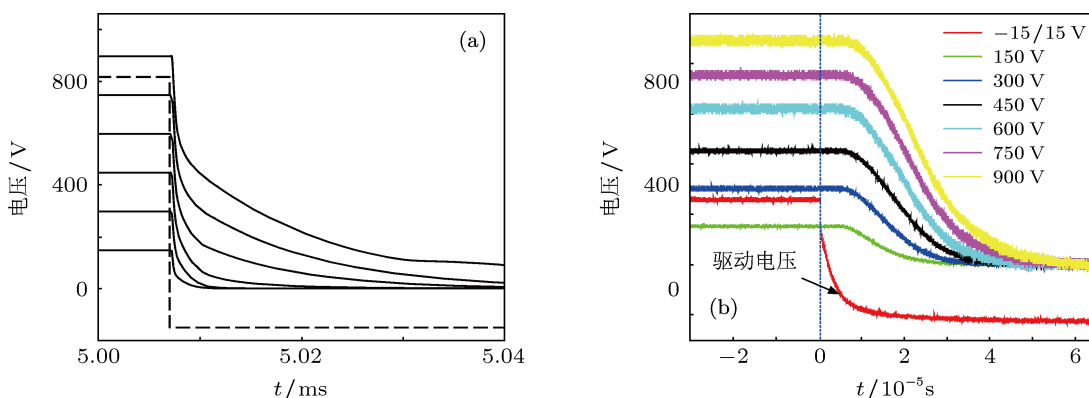
图 5 电流 0.6 A 电阻电压仿真与实验关断波形 (a) 仿真波形; (b) 实验波形
