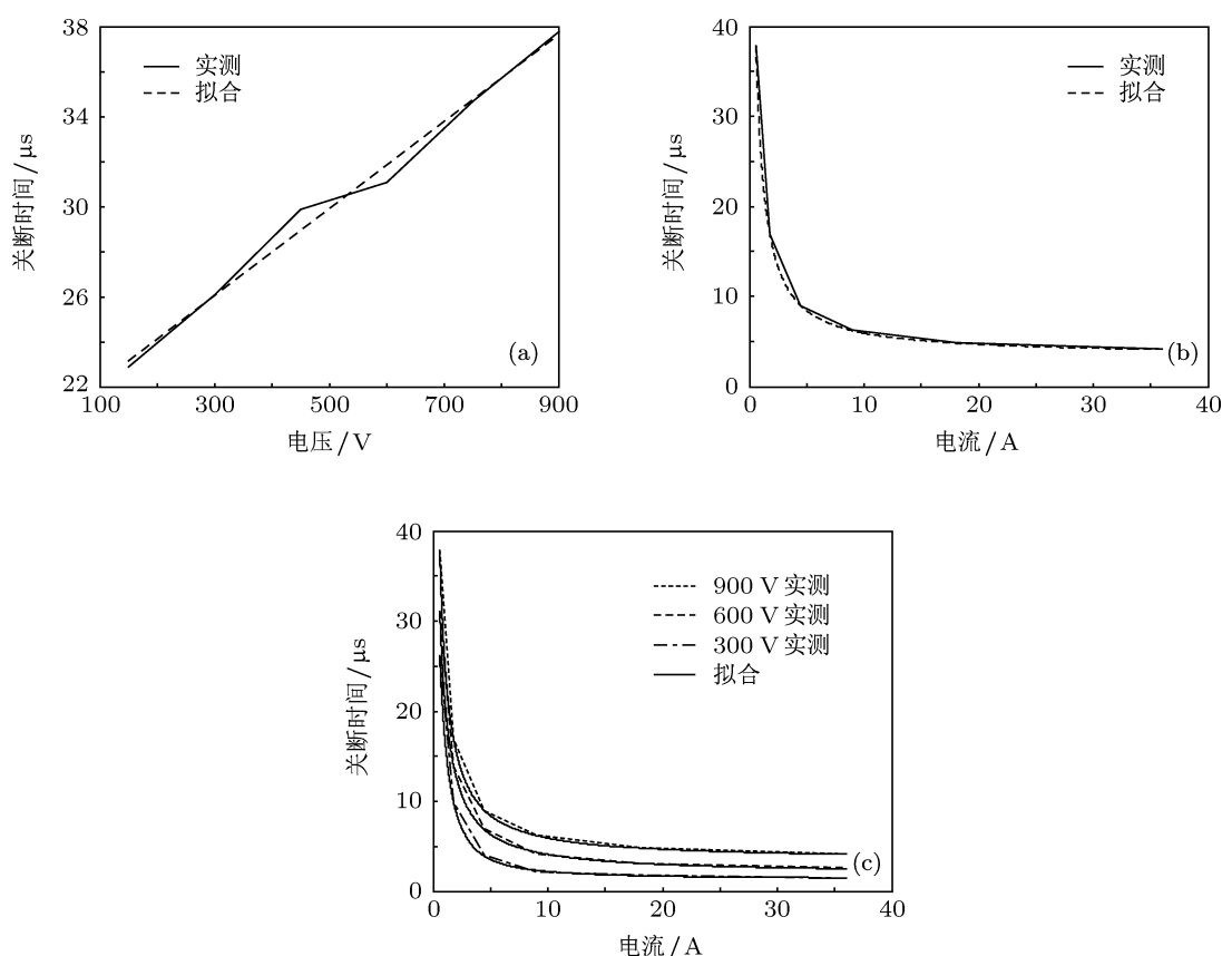
图9 关断时间变化规律 (a) 随电压变化规律; (b) 随电流变化规律; (c) 随电压和电流变化规律
