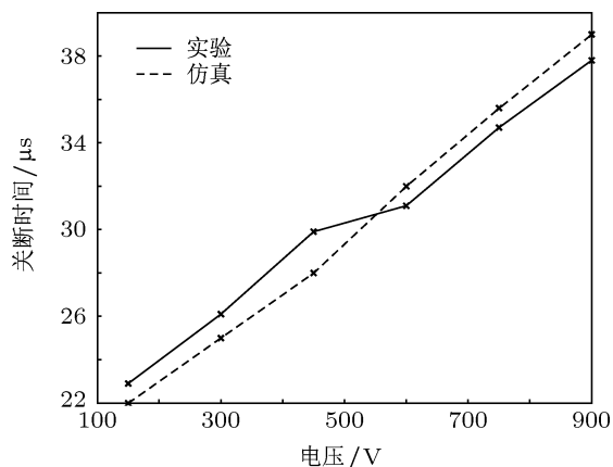
图 6 电流 0.6 A IGBT 关断时间曲线
