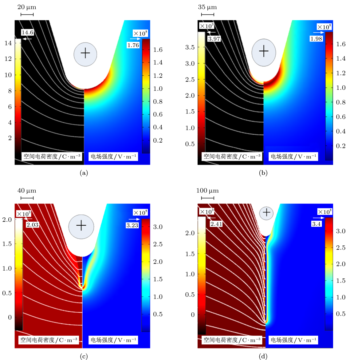
图 5 不同电压幅值下均在 t = 52 ns 时刻电场强度与空间电荷分布 (a) +20 kV; (b) +30 kV; (c) +40 kV; (d) +50 kV
