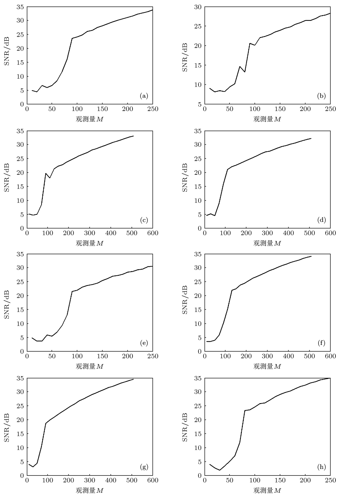
图 4 图像经稀疏采样后重构所得的观测量与信噪比关系及观测量下限阈值 (a) Lena; (b) Yellowstone; (c) Man; (d) Hill; (e) Cameraman; (f) Boat; (g) Barbara; (h) House
