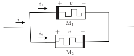
图 6 两个忆阻器反向并联电路
