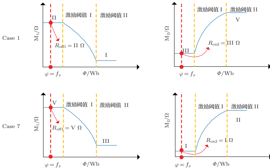
图 14 (网刊彩色) 两种情况下忆阻值和磁通量之间的关系
