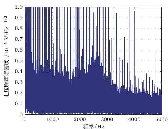
图 7 磁力仪输出电压噪声谱密度, 50 Hz 的谐波来自于工频干扰
