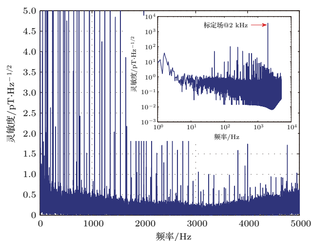
图 8 磁力仪灵敏度, 图中插图为对数坐标表示
