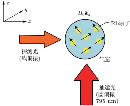
图1 (网刊彩色) 磁力仪光场配置示意图
