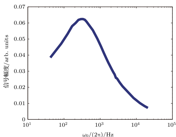
图 6 信号幅度随 \omega_0 的变化
