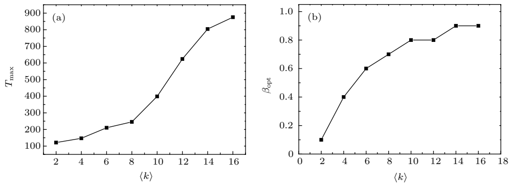
图3 (a) 网络最大生存时间 T_{\max} 及其 (b) 最佳参数 \beta_{\text{opt}} 与网络平均度 \langle k \rangle 的关系
