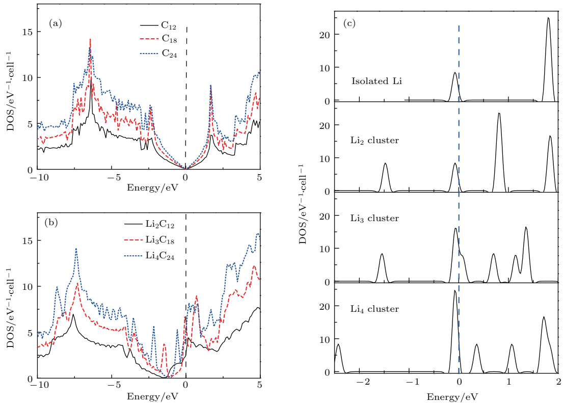
图2 (网刊彩色) (a) 石墨烯 (C 12 , C 18 , C 24 ) 的态密度图; (b) 对应图 1(a) 中石墨烯吸附 Li 团簇 (Li 2 C 12 , Li 3 C 18 , Li 4 C 24 ) 的态密度图; (c) 孤立 Li 原子, Li 2 , Li 3 , Li 4 团簇的态密度图
