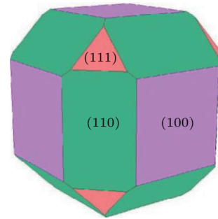
图 6 (网刊彩色) 由 Wulff 定理截成的多面体 Fig. 6. (color online) A polyhedron truncated by the Wulff theorem.
