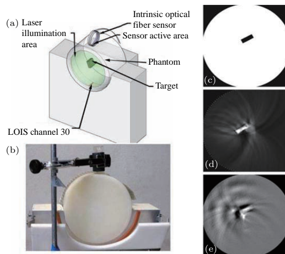
图 15 (a) 样品固定装置结构示意图; (b) 样品固定装置实物图; (c) 样品内部结构示意图; (d) 压电换能器成像图; (e) 光纤传感器成像图; 引自文献 [4]
