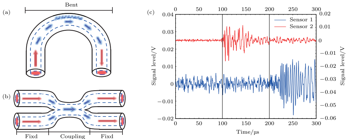
图2 (a) 光纤弯曲损耗型超声传感结构; (b) 光纤耦合损耗型超声传感结构; (c) 光纤耦合损耗型超声传感器时域响应; 引自文献 [48—54]
