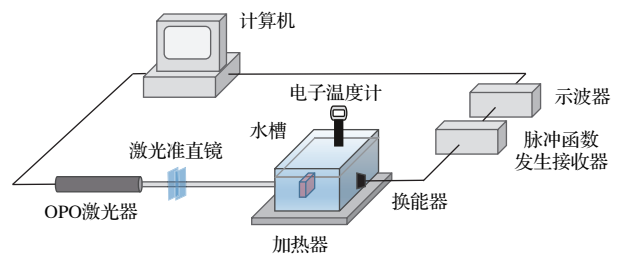
图1 实验系统结构示意图
