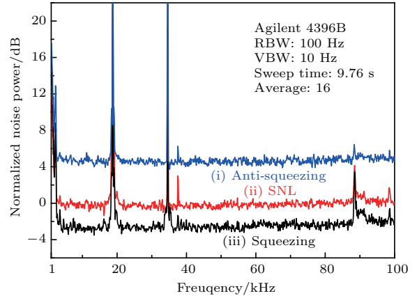
图4 利用量子噪声锁定技术后得到的压缩谱 分析频率 1—100 kHz; RBW 100 Hz; VBW 10 Hz, 在 2.6—100 kHz 的分析频率范围内得到了 -2.8 dB 的压缩, 其中电子学噪声已经被扣除 Fig. 4. Noise spectra with the quantum noise locking method. Analysis frequency, 1—100 kHz; RBW, 100 Hz; VBW, 10 Hz, squeezing level of -2.8 dB is obtained at 2.6—100 kHz. Electronic noise has been subtracted.
