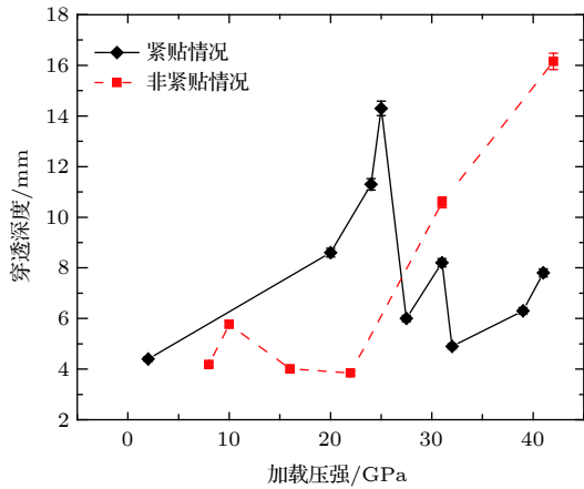
图 7 紧贴条件和非紧贴条件下, 不同压强下微喷颗粒在泡沫中的穿透深度比较 Fig. 7. Penetration depth of the tin fragments in foam versus pressure, with and without vacuum gap.
